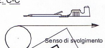
Sez. C-C
