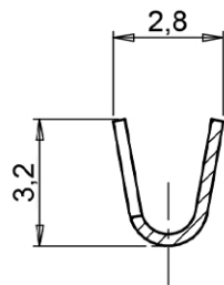
SEZ. A-A
